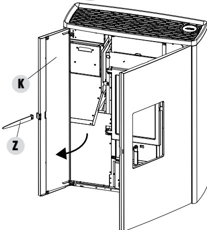
KLAPPE FÜR DIE PELLET-BESCHICKUNG „K“
