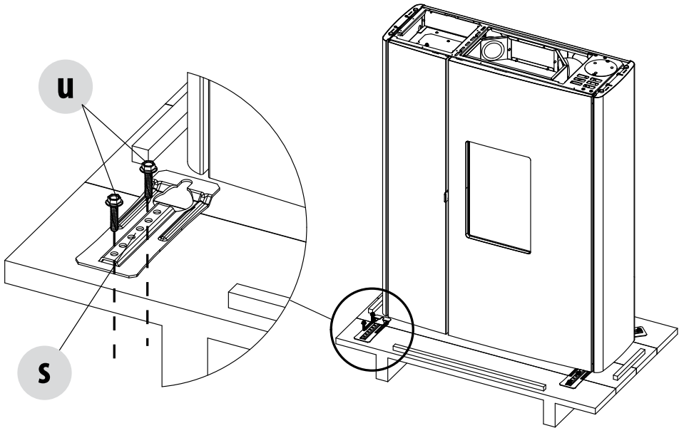
ENTFERNUNG DER BEFESTIGUNGSBÜGEL
