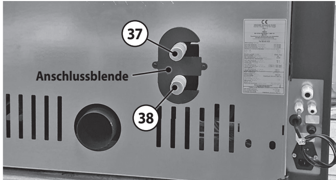
(Die obige Abbildung zeigt die Anschlüsse Rücklauf (38) und Vorlauf (37) mit aufgesetzten Transport-Schutzkappen)
