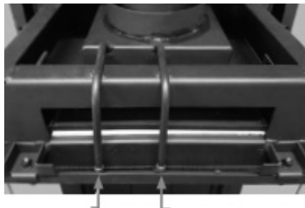
Abb. 3.4 Messöffnungen, links Verbrennungsluft (Ringspalt); rechts Abgasanalysemessung
