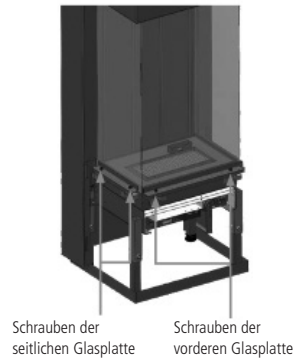
Abb. 2.5 + Abb. 2.6 Lösen Sie die 4 Schrauben (2 oben, 2 unten), entfernen Sie sie jedoch nicht.
