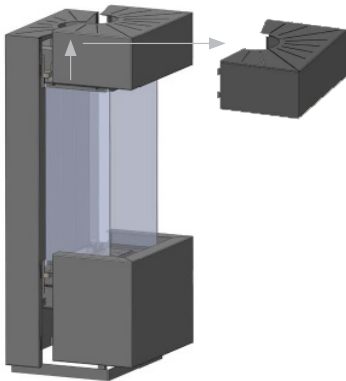
Abb. 3.1 Entfernen der oberen Abdeckung
