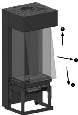
Abb. 2.6 Heben Sie die Glasscheibe vorsichtig bis zum Anschlag an; die Glasscheibe kann sich nicht aus der Nut lösen. Anschließend kann man die Scheibe schräg nach unten ziehen. Stellen Sie das Glas an einem sicheren Ort ab, damit es nicht herunterfällt und/oder beschädigt wird:
