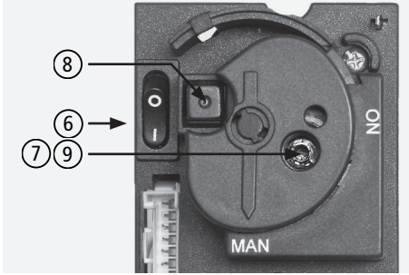
Abb. 5.20 Hauptschalter der Steuer- und Reglereinheit ausschalten
