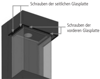
Abb. 2.5 + Abb. 2.6 Lösen Sie die 4 Schrauben (2 oben, 2 unten), entfernen Sie sie jedoch nicht.
