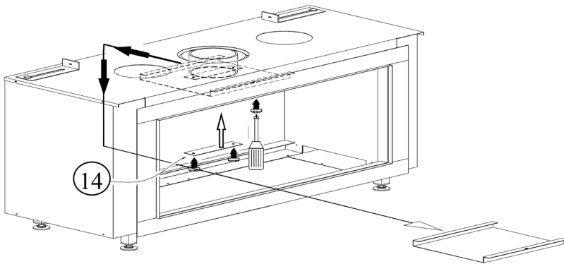
Abb. 6.2 Drosselscheibe und Prallplatte
