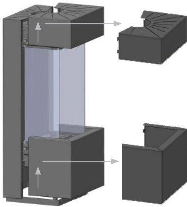
Abb. 2.3 Entfernen Sie die oberen und unteren Abdeckungen vom Mantel. Diese sind mit 4 Haken pro Abdeckung befestigt. Schieben Sie die Abdeckung zuerst nach oben und ziehen Sie das Unterteil nach außen. Sowohl die obere als auch die untere Abdeckung können entfernt werden.
