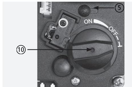
Abb. 5.21 Stellknopf des Gasreglers
