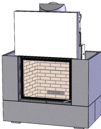
Abb. 4: Bauteile des zweiten Rings setzen
