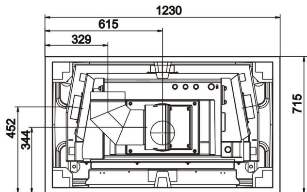
Abb. 15: Rauchgasabgang hinten
