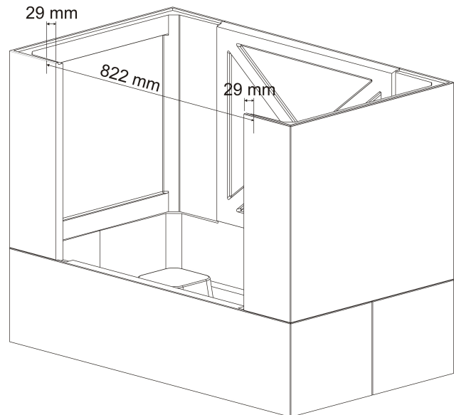
Abb. 14: Nachbearbeitung für Kamin-Kessel 62/76 Drehtür
