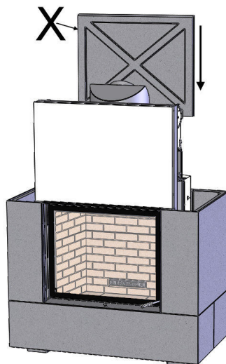
Abb. 5: Rückwandplatte (X) einsetzen (entfällt bei der Tunnel-Variante)
