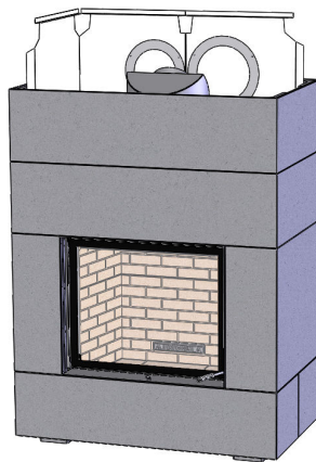
Abb. 8: Vierten Ring aufsetzen
