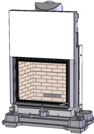
Abb. 2: Posez le foyer Stil-Kamin sur la plaque de base et ajustez lui
