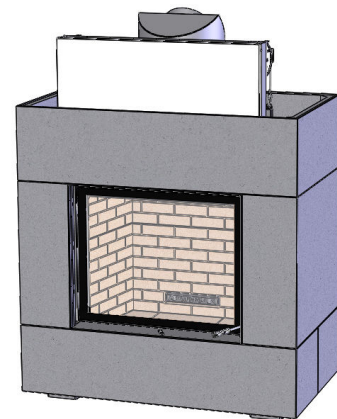
Abb. 6: Dritten Ring aufsetzen
