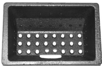
Fig. 35 - Beispiel einer sauberen Brennschale
