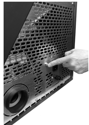
Fig. 34 - Manueller Reset
