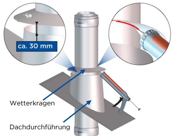
Bild 5-26: Dachdurchführung
