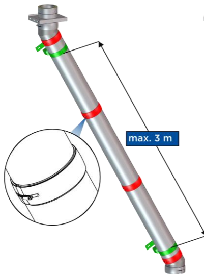
Bild 5-23: Schrägföhrung 30°
