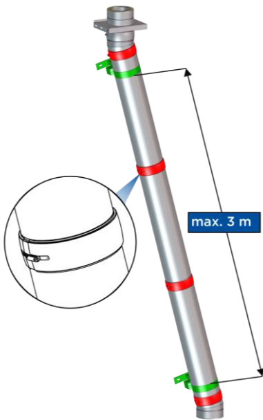
Bild 5-22: Schrägföhrung 15°
