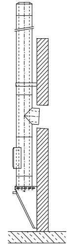
Bild 5-4: Aufbau Grundplatte mit Kondensatablauf und Konsolblech „schenkelabwärts“
