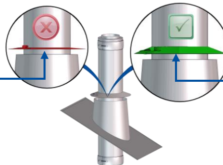
Bild 5-27: Befestigung Wetterkragen
