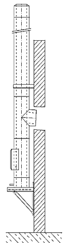
Bild 5-5: Aufbau Grundplatte mit Kondensatablauf und Wandstütze „schenkelabwärts“
