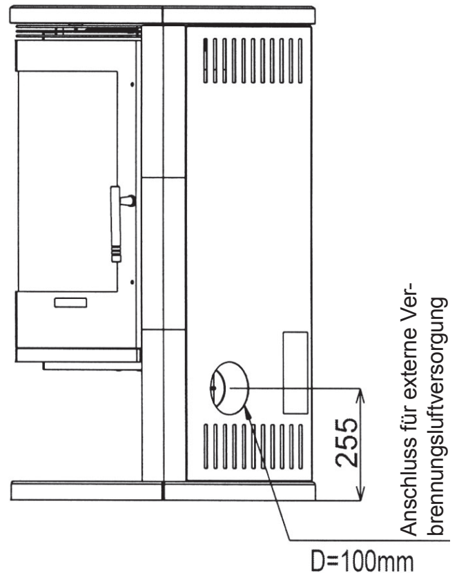
Abb. 1 Obere Rauchrohröffnung
