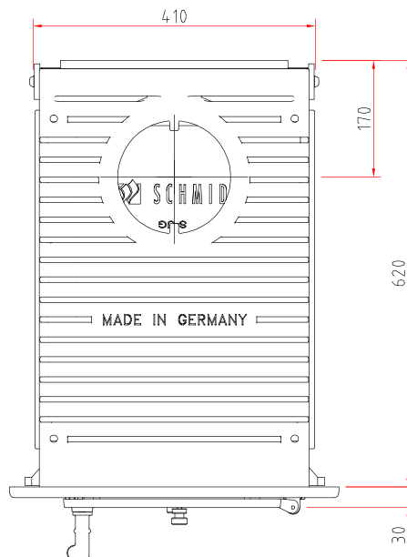
Draufsicht M 1:10
